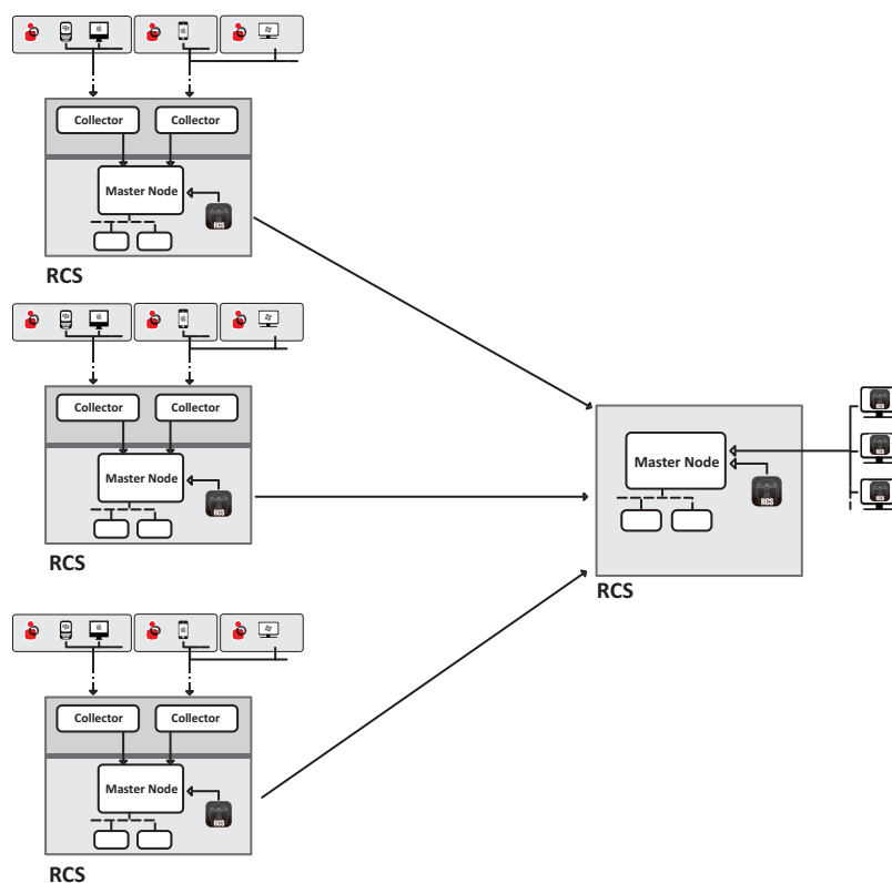
Figura 2: Architettura RCS multi a uno: schema logico
