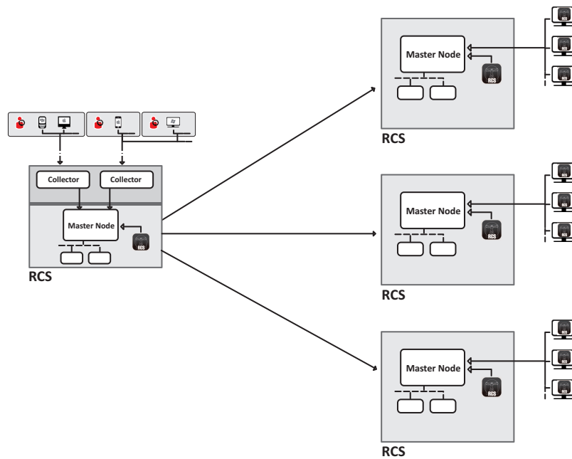
Figura 1: Architettura RCS uno a molti: schema logico
