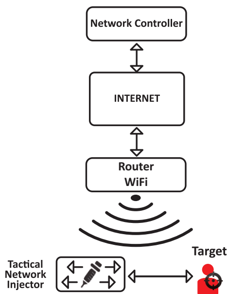
Figura 1: Tactical Network Injector: schema di collegamento standard
