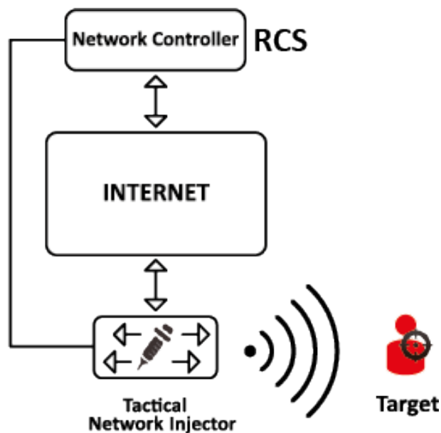
Figura 2: Tactical Network Injector: schema in emulazione di access point
