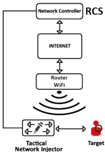
Figura 1: Tactical Network Injector: schema di collegamento standard
