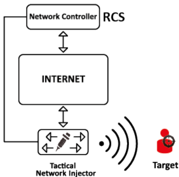
Figura 2: Tactical Network Injector: esquema de emulación de punto de acceso
