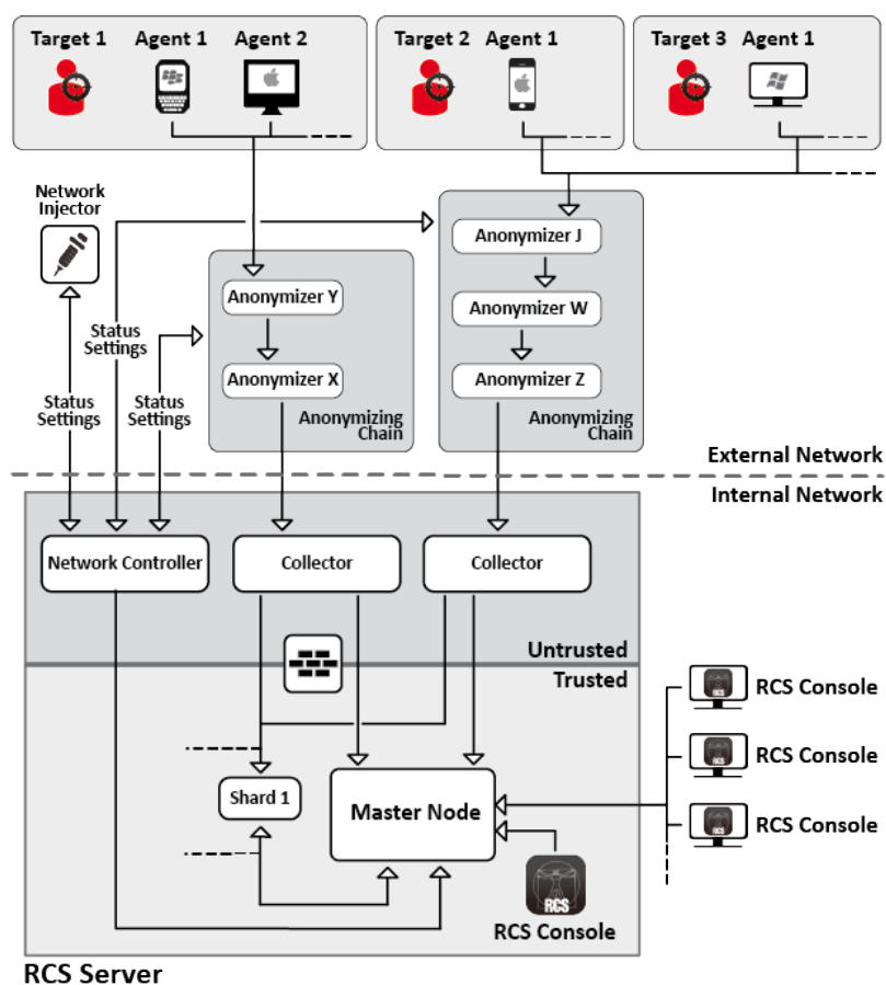
Figura 1: Arquitectura de RCS: esquema lógico
