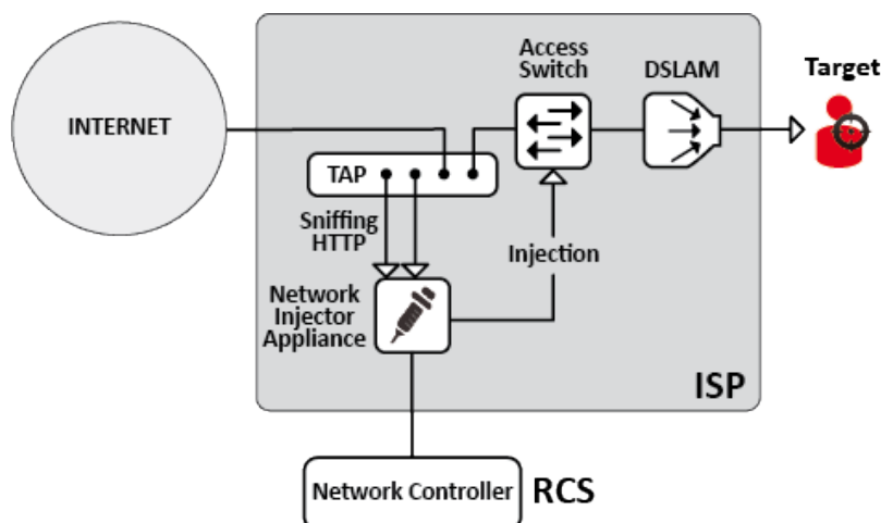
Figura 2: Network Injector Appliance con TAP: esquema físico
