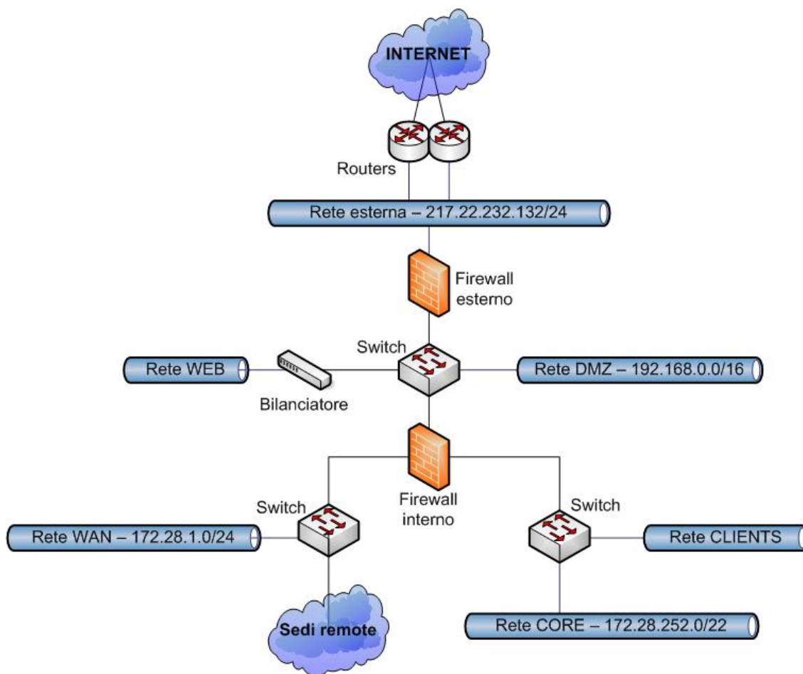
Figura 1 - Schema di massima delle interconnessioni di rete
