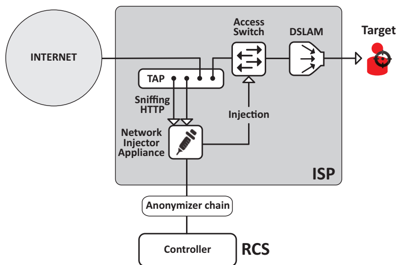
Figura 2: Network Injector Appliance con TAP: schema fisico
