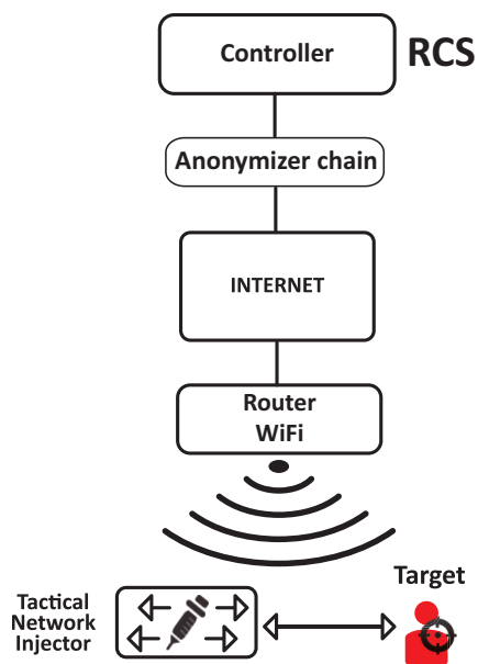
Figura 1: Tactical Network Injector: schema di collegamento standard
