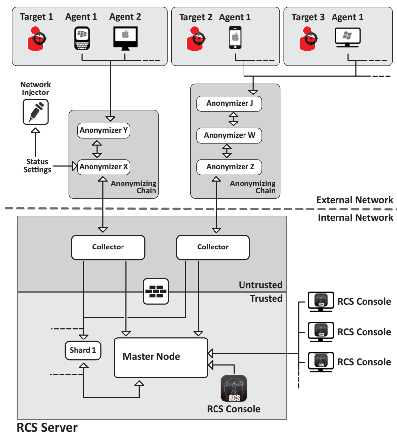
Figura 1: Architettura RCS: schema logico
